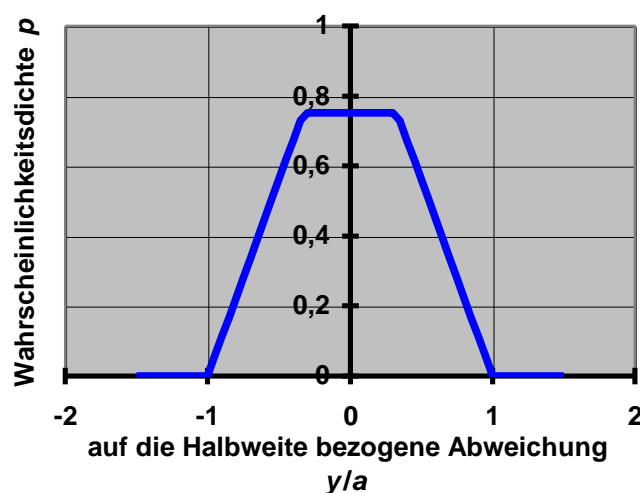
Bild 1: Auf die Halbweite bezogene symmetrische trapezförmige Wahrscheinlichkeitsdichte mit dem Wert \beta = 0,33 des Knickpunktparameters, die sich aus der Faltung von zwei Rechteckverteilungen ergibt.
